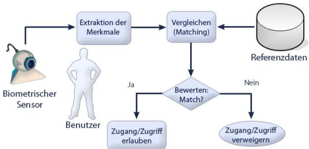
Abbildung 7: Schematische Darstellung einer biometrischen Zugangs-/Zugriffskontrolle
