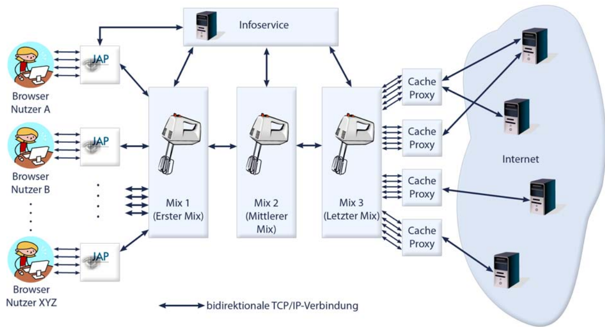
Abbildung 10: Grobarchitektur von AN.ON
