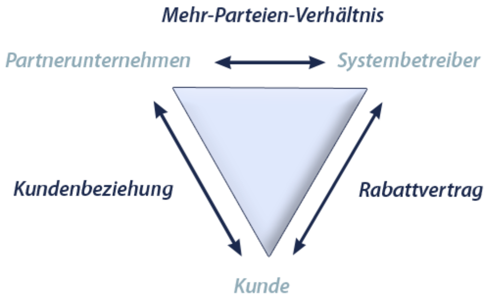
Abbildung 5: Mehr-Parteien-Kundenbindungssystem
