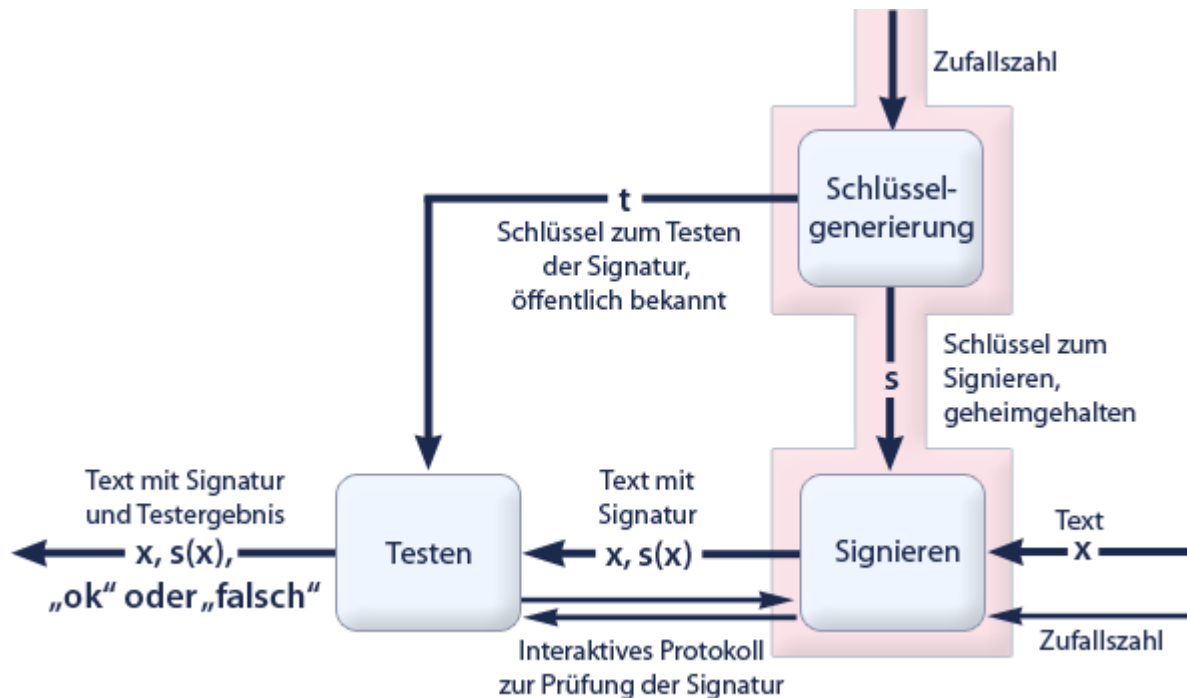
Abbildung 12: Digitales Signatursystem für nicht herumzeigbare Signaturen
